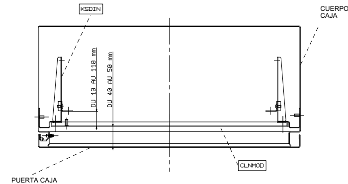
VISTA SECCIÓN CAJA CON ACCESORIOS
